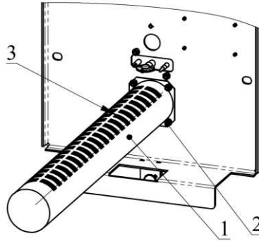
1 - газовый рожок, 2 - винт М5, 3 - отверстия рожка. Рисунок - 3 Установка газового рожка.
