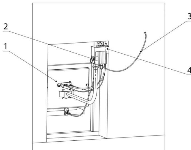
1 - капилляр термостата, 2 - термостат, 3 - кронштейн, 4 - винт. Рисунок - 5 Установка термостата.
