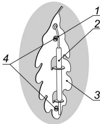
1. Капельяр термостата, 2. Термостат, 3. Кронштейн, 4. Винт Рисунок 5. Установка термостата
